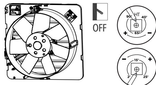
EASY 15/6 A HT - EASY 23/9 AR HT - EASY 30/12 AR HT
