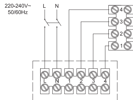
EASY 15/6 A T - EASY 23/9 AR T - EASY 30/12 AR T
