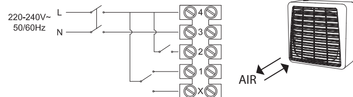
EASY 23/9" AR T/HT - EASY 30/12" AR T/HT ASPIRAZIONE/VENTILAZIONE - EXTRACT/INTAKE
