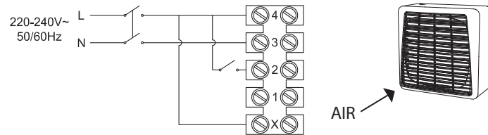
EASY 23/9" AR T/HT - EASY 30/12" AR T/HT SOLO VENTILAZIONE - INTAKE ONLY
