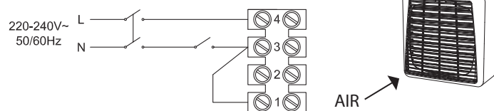
EASY 23/9" AR - EASY 30/12" AR SOLO ASPIRAZIONE - EXTRACT ONLY
