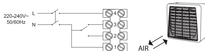
EASY 23/9" AR - EASY 30/12" AR ASPIRAZIONE/VENTILAZIONE - EXTRACT/INTAKE
