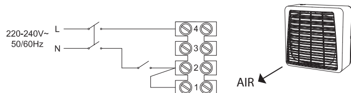
EASY 23/9" AR - EASY 30/12" AR SOLO VENTILAZIONE - INTAKE ONLY
