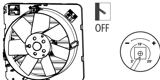
EASY 15/6 A HT - EASY 23/9 AR HT - EASY 30/12 AR HT
