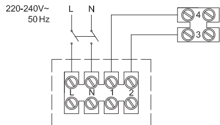
EASY 23/9" AR - EASY 30/12" AR SOLO ASPIRAZIONE - EXTRACT ONLY
